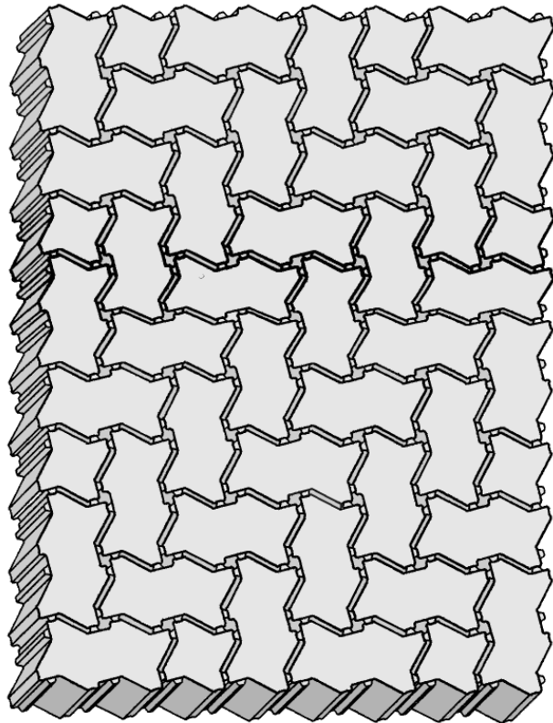
Drain-Maxima Verlegemuster
